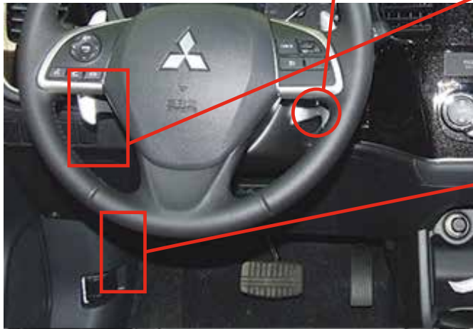
② ⑤ ⑥ Harness in Driver kick panel, close to fire wall Harnais dans le panneau latéral côté conducteur, prêt du pare-feu
