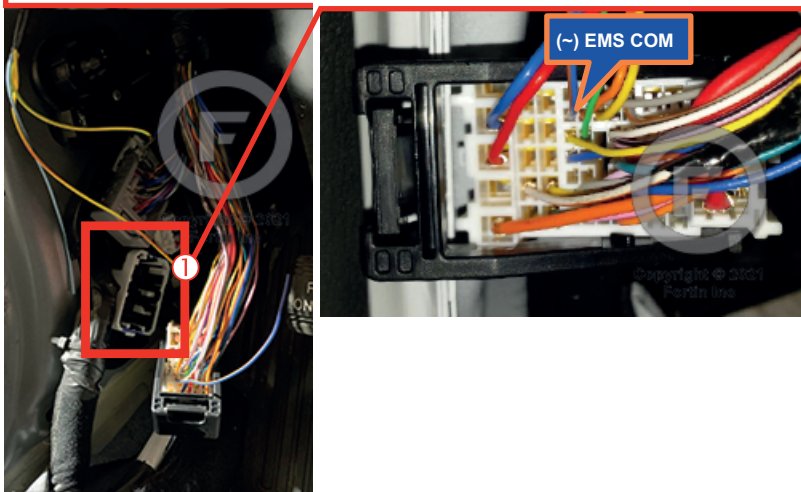
① Driver Kick Panel Panneau latéral côté conducteur
