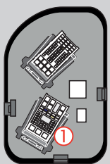
1 Back view 58-pin White or Red connector Driver kick Panel Vue de dos Connecteur Blanc ou Rouge de 58 pins Panneau latéral côté conducteur
