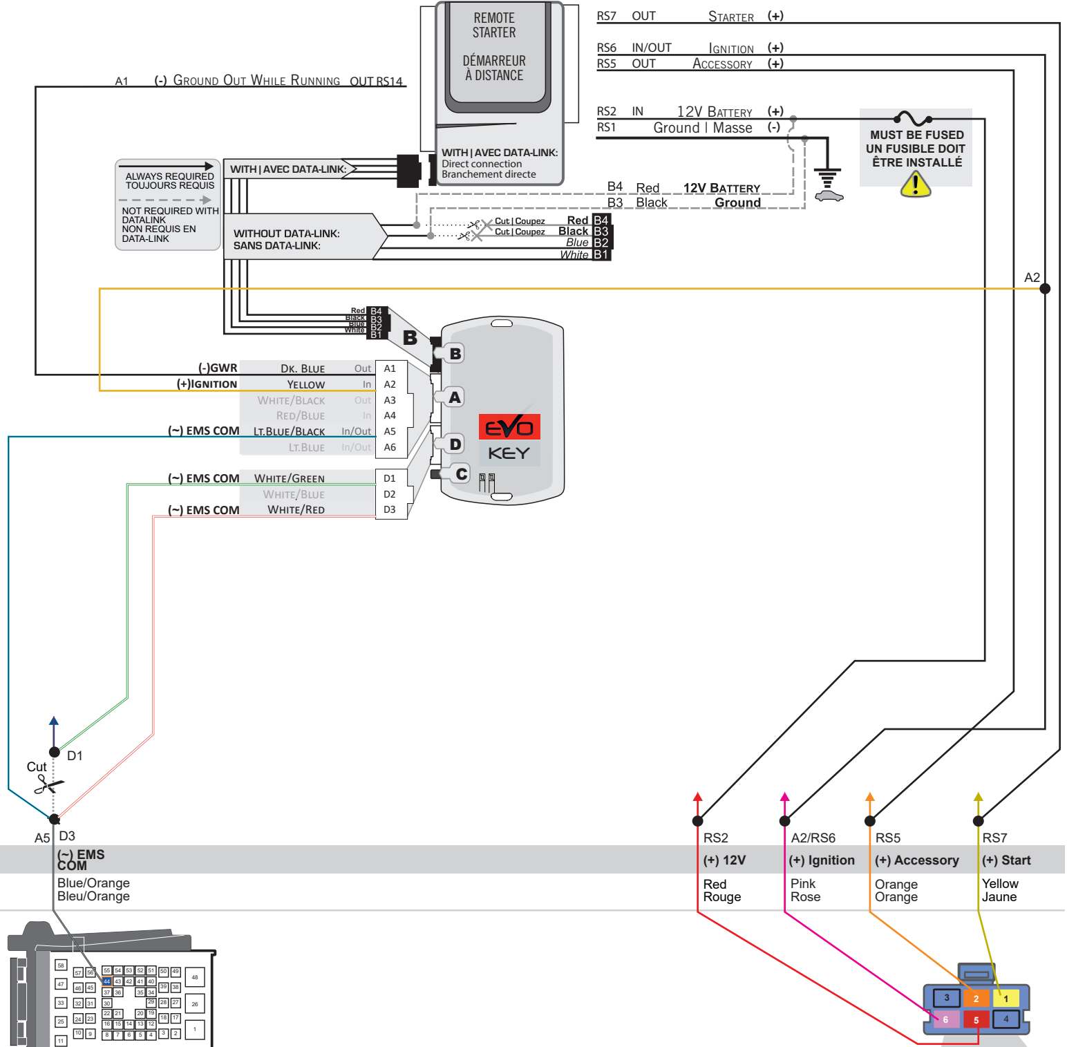
1 Back view 58-pin White or Red connector Driver kick Panel Vue de dos Connecteur Blanc ou Rouge de 58 pins Panneau latéral côté conducteur
