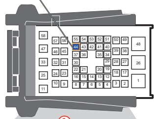
1 Back view 58-pin White or Red connector Driver kick Panel Vue de dos Connecteur Blanc ou Rouge de 58 pins Panneau latéral côté conducteur
