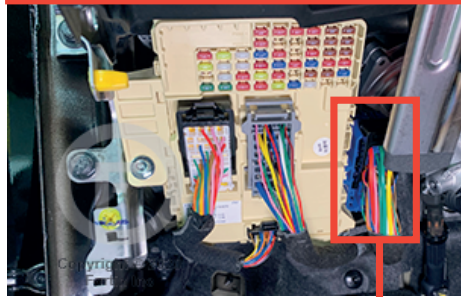
1 Right side of fusebox À la droite de la boîte à fusibles
