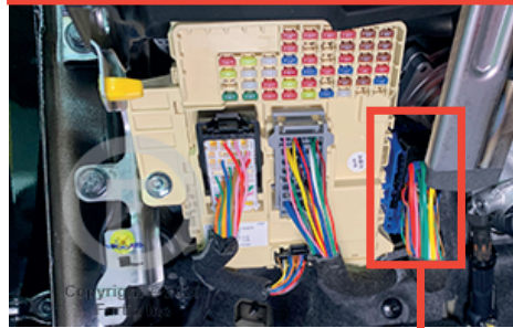
① Right side of fusebox À la droite de la boîte à fusibles
