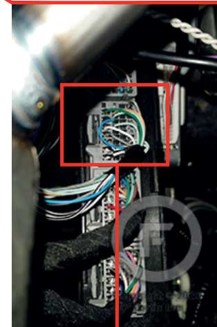
④ Hybrid ECU, Left of the steering colum. ECU Hybride, Côté conducteur, à gauche de la colonne de direction.
